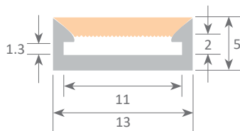
Scale 1:2
